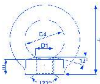
DIN 582 Eyenuts
