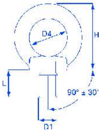
DIN 580 Eyebolts
